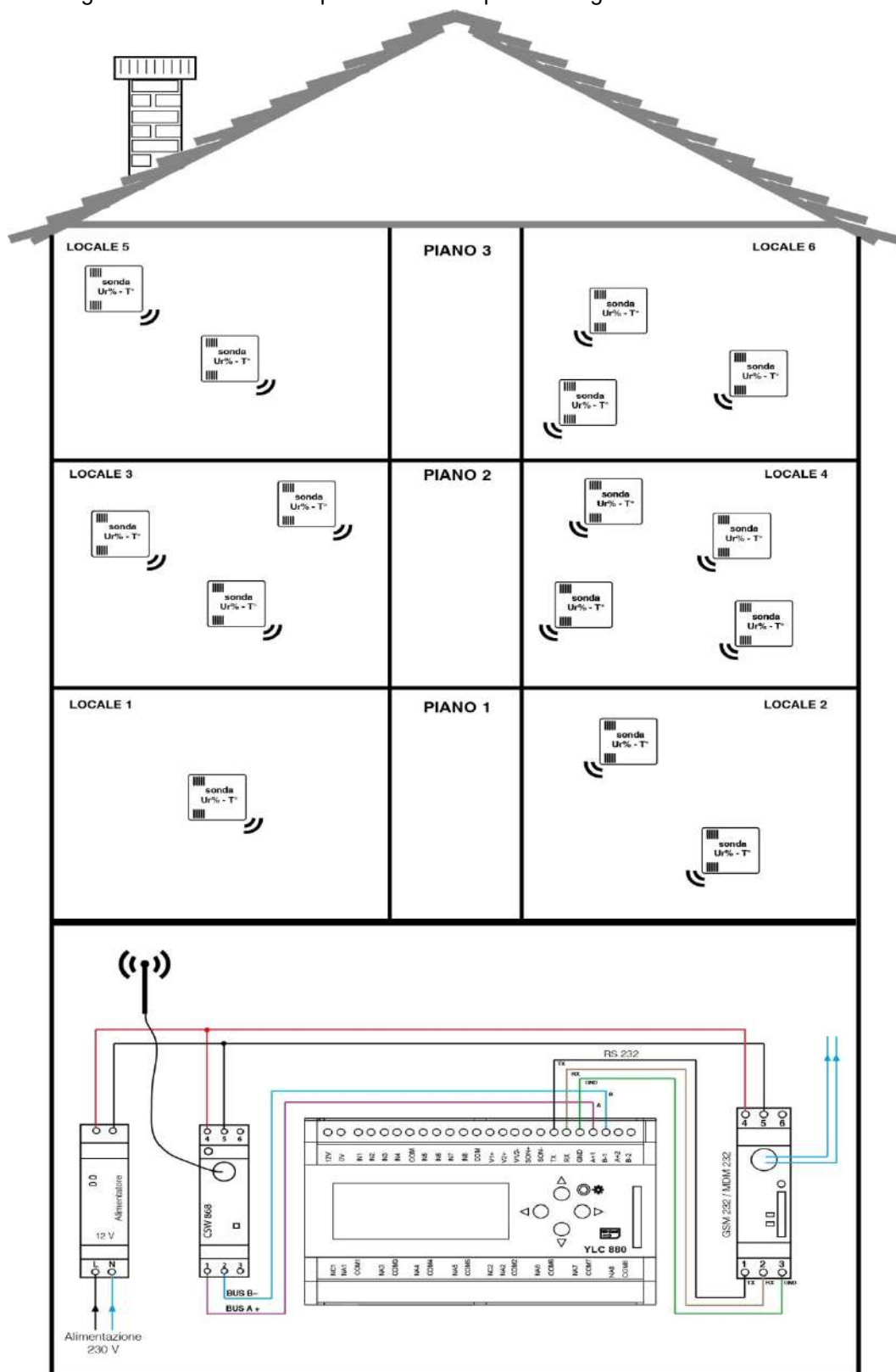
Esempio 1: rete con sonde wireless
